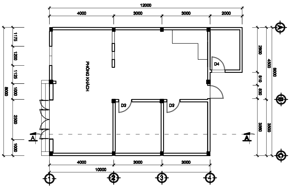
MẶT BẰNG TẦNG 1 (TL 1:100)
