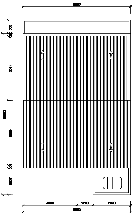
MẶT BẰNG MÃI ( TL 1:100)
