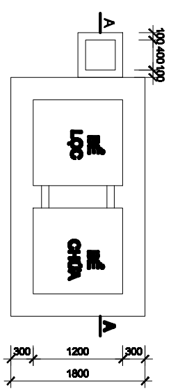
HẦM TỰ HOẠI (TL 1:50)
