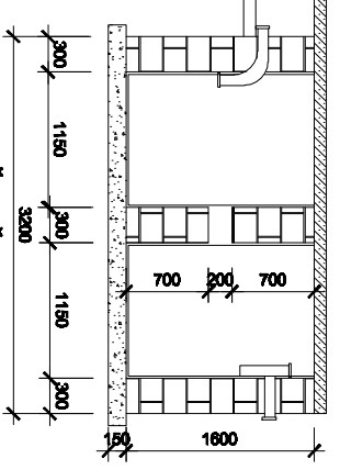
HẦM TỰ HOẠI (TL 1:50)
