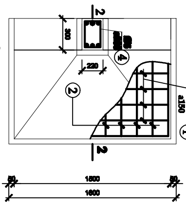
MÔNG MBT (TL 1:25)
