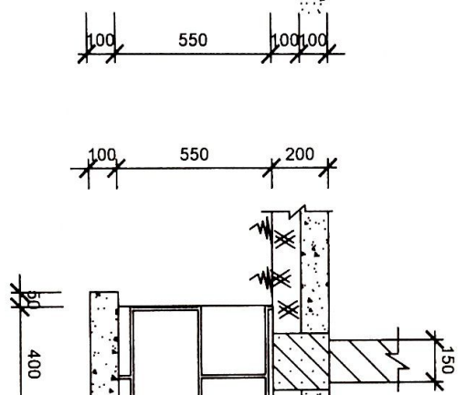
MÔNG M2 ( TL : 1:25 )
