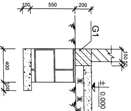
MÔNG M1 ( TL : 1:25 )
