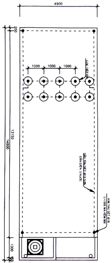
MẶT BẰNG HỆ THỐNG CHỒNG SÉT ( TL 1:100)
