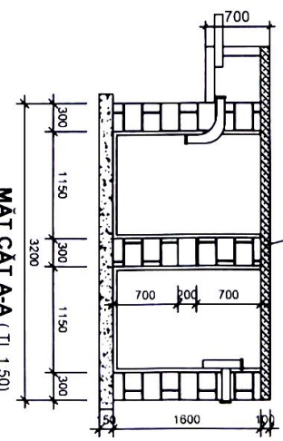
MẶT CẮT A-A (TL 1:50)
