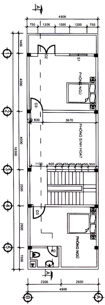
MẶT BẰNG TẦNG 2 ( TL 1:100)
