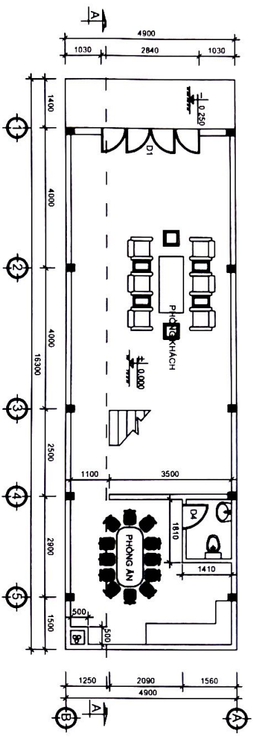
MẶT BẰNG TẦNG 1 ( TL 1:100)
